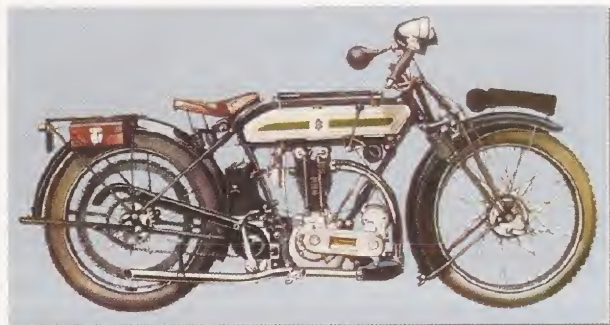
Motocicleta Triumph-500-Ricardo (1924)
